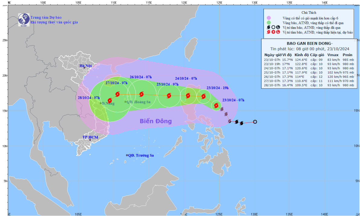
Hình 1: Bản đồ dự báo quỹ đạo và cường độ bão Trami phát lúc 08 giờ, ngày 23/10/2024.
